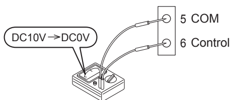
[Abb. 9] Spannung des Mischventils (Steuerung)
