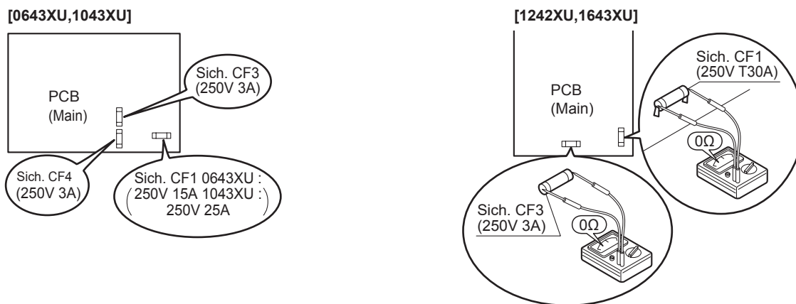
[Abb. 1] Stromdurchfluss der Sicherung an PCB (Main)
