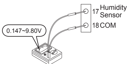
[Abb. 7] Spannung des Feuchtigkeitsensors
