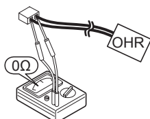
[Abb. 10] Widerstand des Relais der den Kompressor vor Überhitzung schützt (OHR).
