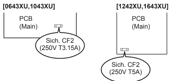
[Abb. 6] Stromdurchgang der Sicherung an der PCB (Main)
